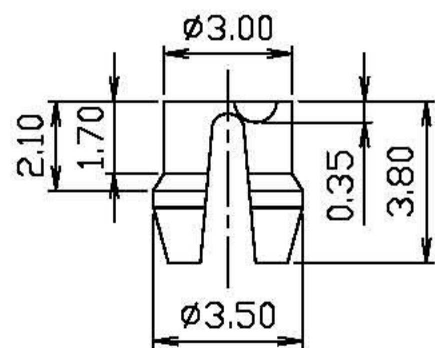
DETAIL Y
