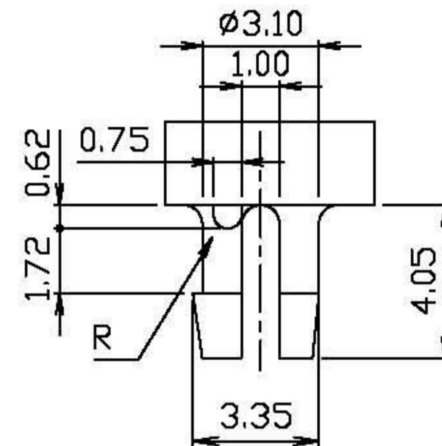
DETAIL Y
